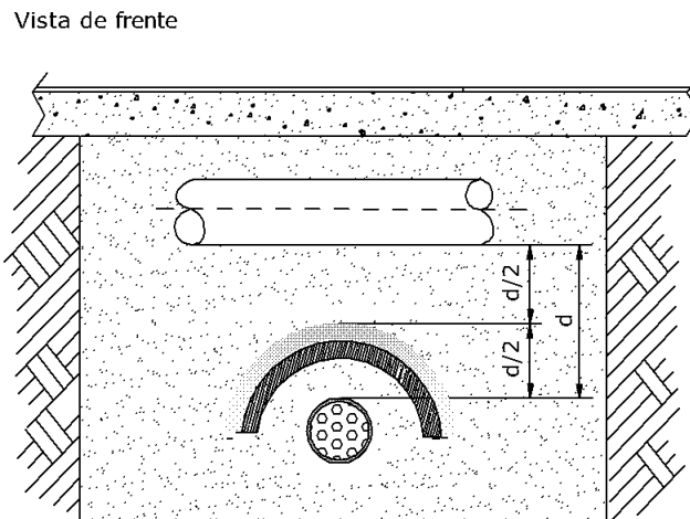
Figura 6b Protección con media caña o media caña de PE/PVC/PP/PRFV más planchas de caucho sintético Cruce
