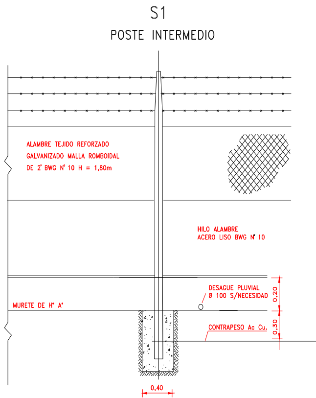
POSTE INTERMEDIO
