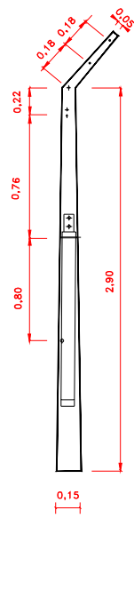
POSTE TENSOR
